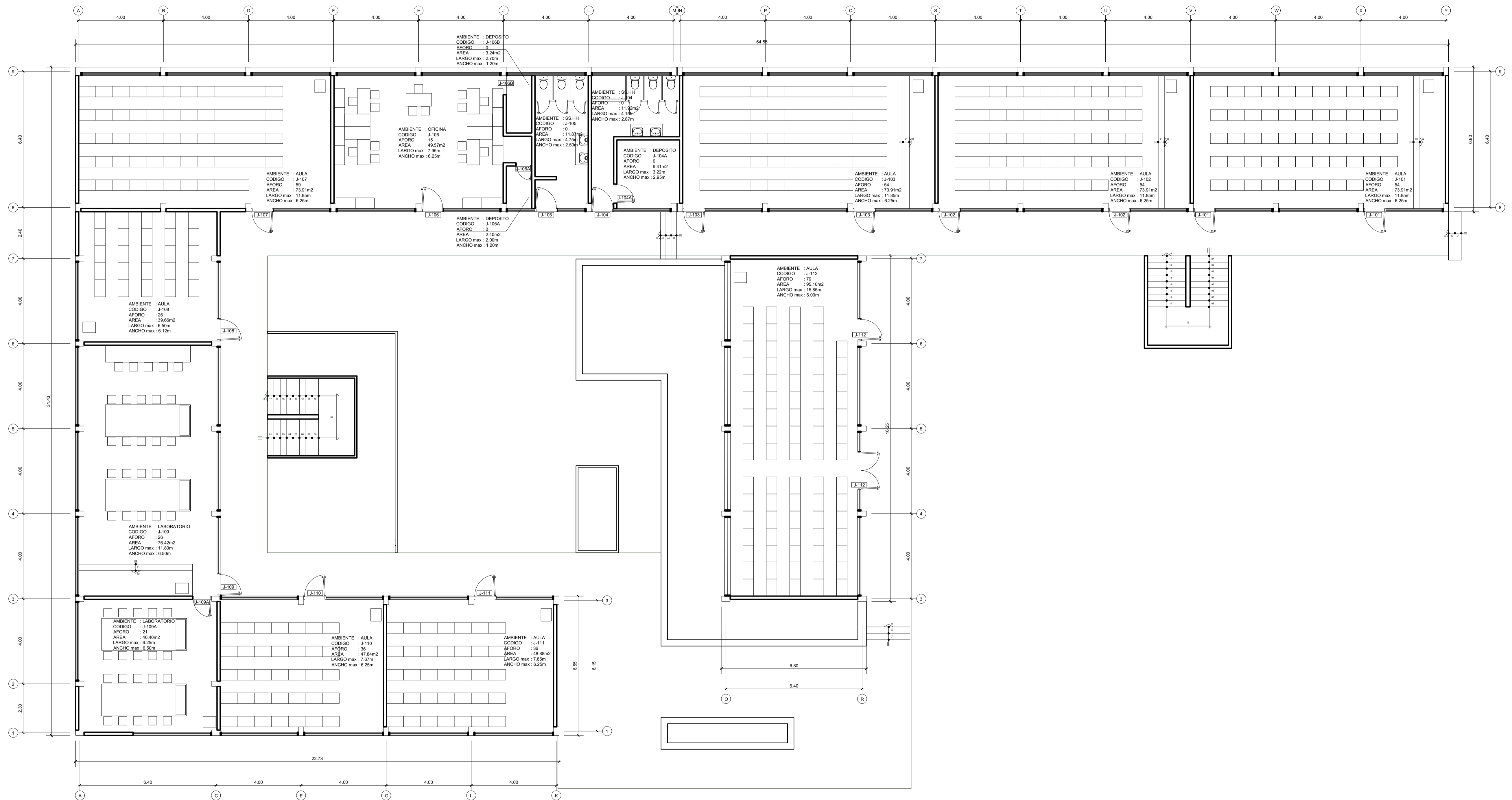
PRIMERA PLANTA AREA TECHADA = 1046.37m 2 AFORO = 460 ESCALA 1:100
